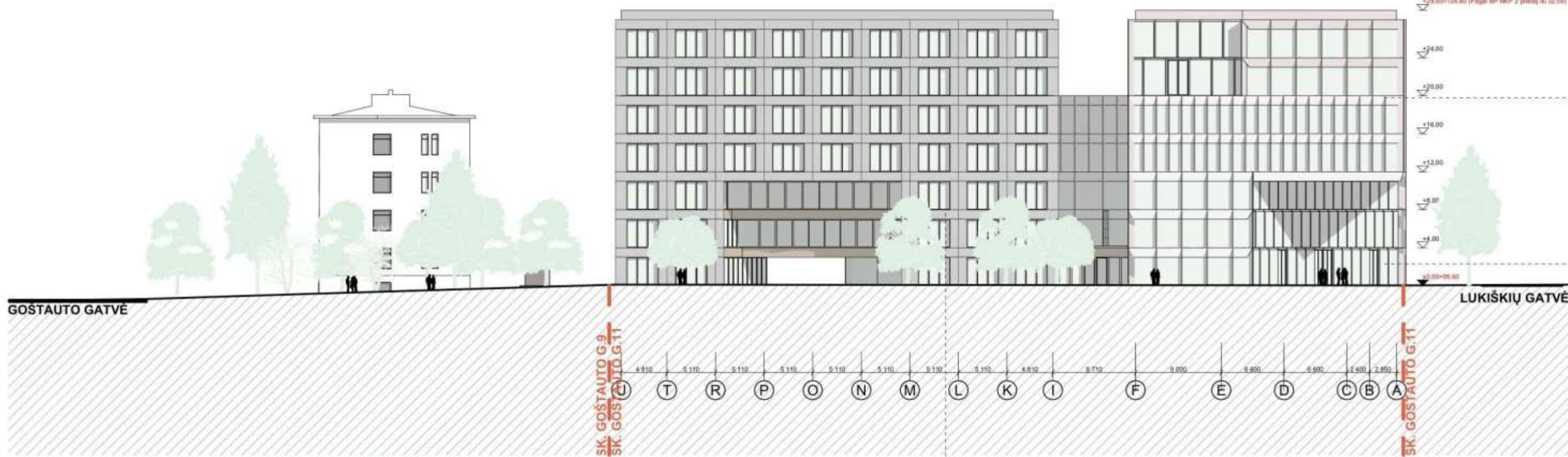
UPĖS ALĖJOS IŠKLOTINĖ. VIDUTINĖ ŽEMĖS ALTITUDĖ + 95,60.
