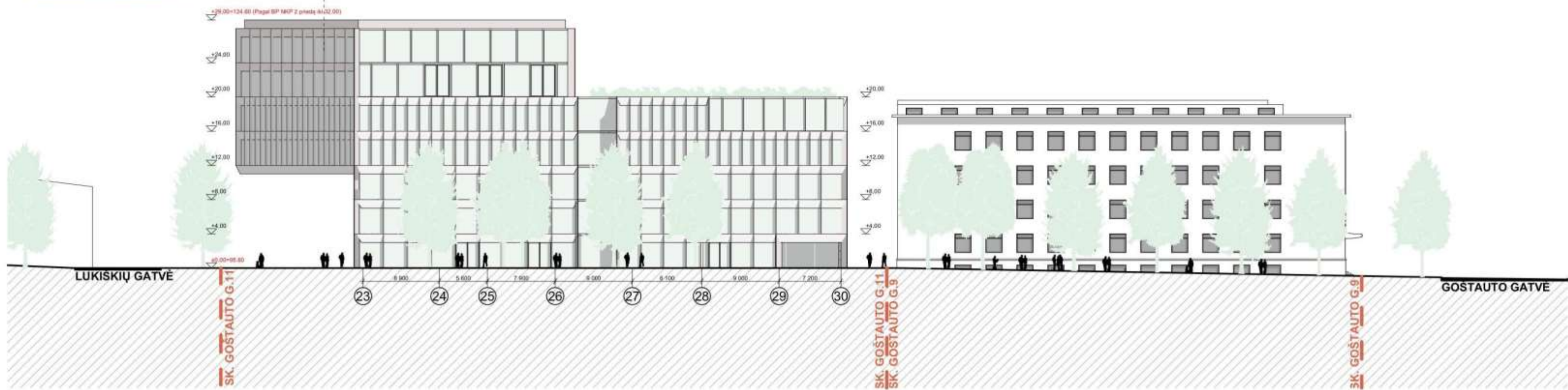
MEČETĖS GATVĖS IŠKLOTINĖ. VIDUTINĖ ŽEMĖS ALTITUDĖ + 95,60.
