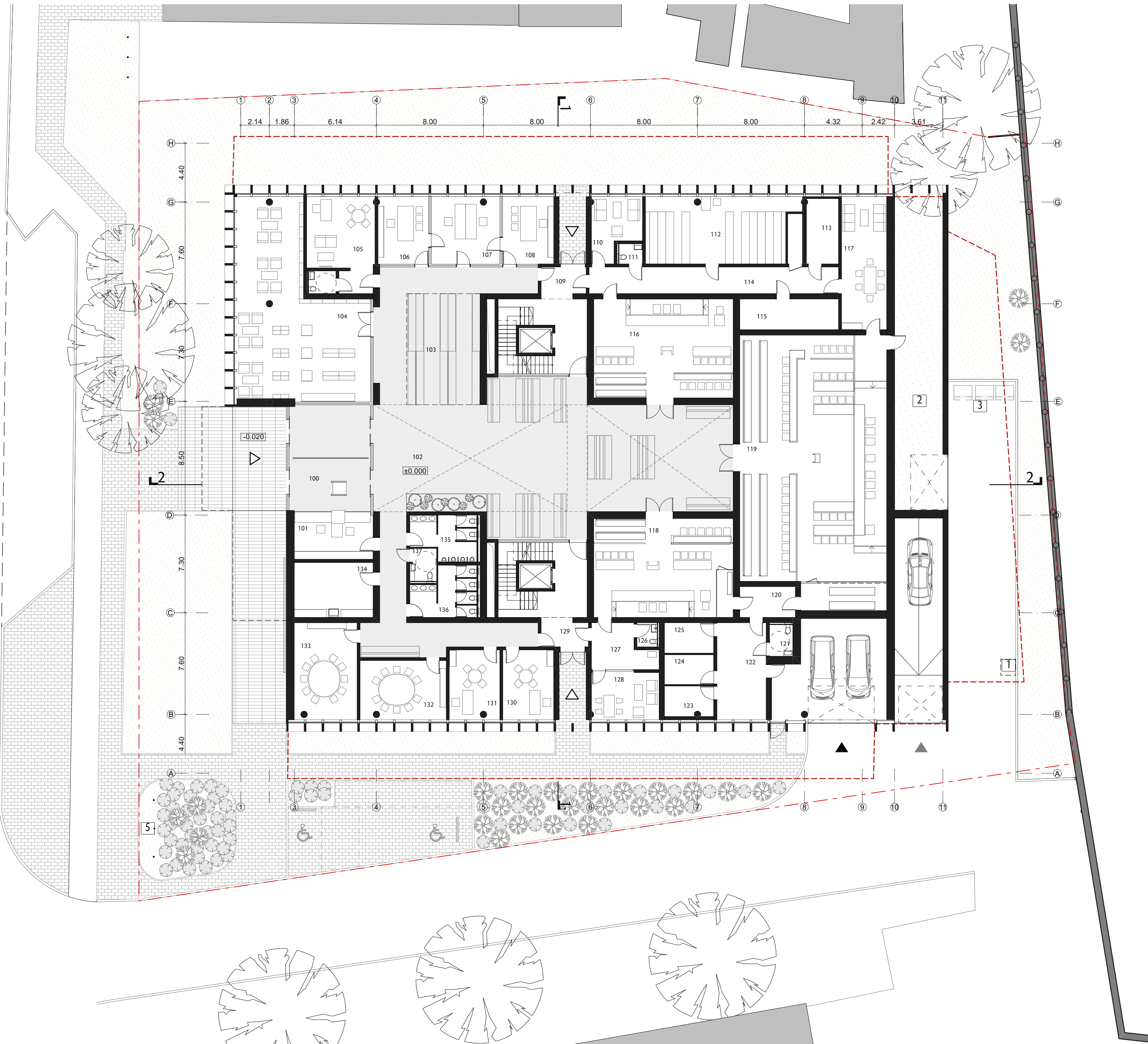
PIRMO AUKŠTO PLANAS M 1:200
