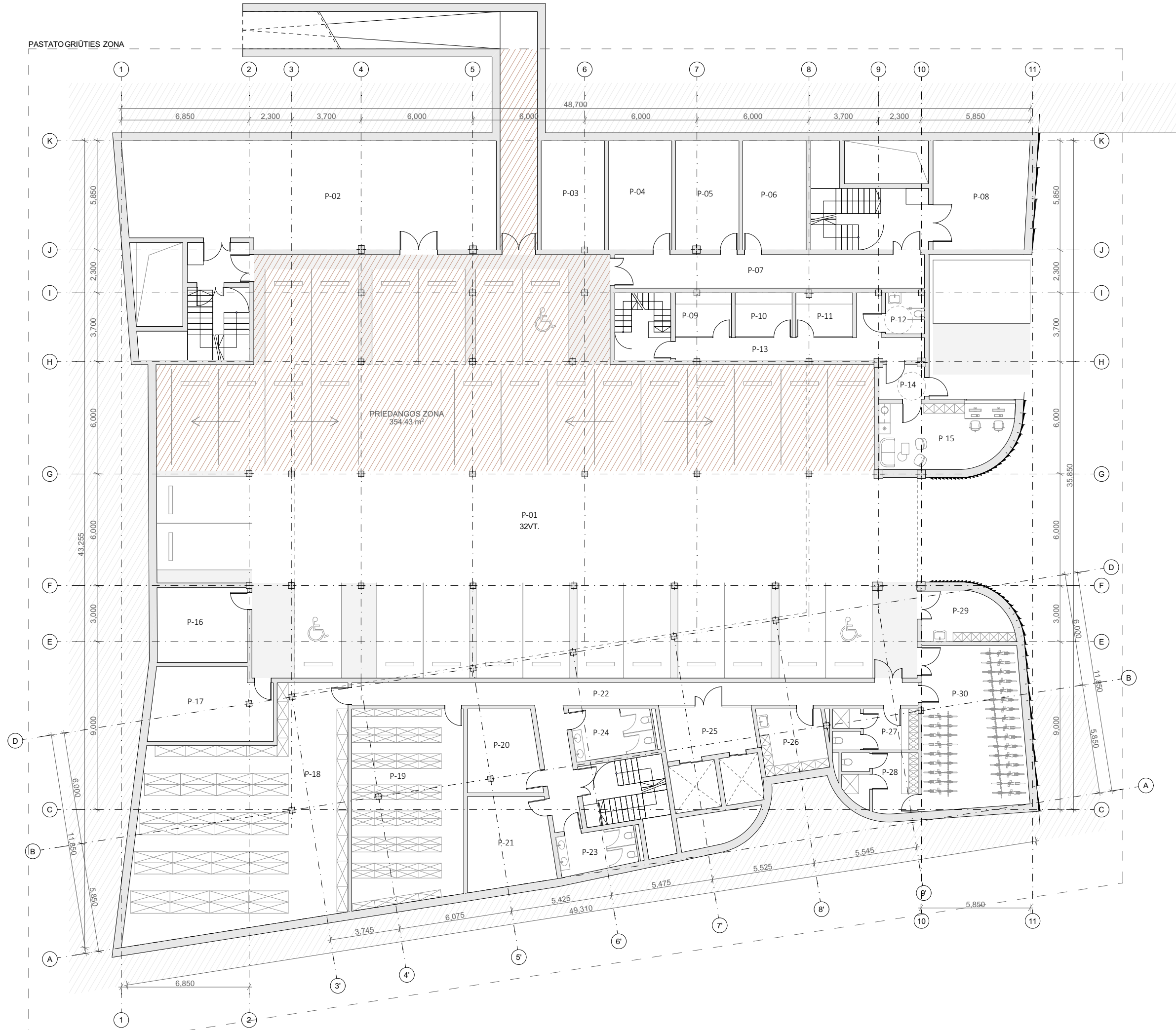
-1 AUKŠTO PLANAS M1:200
