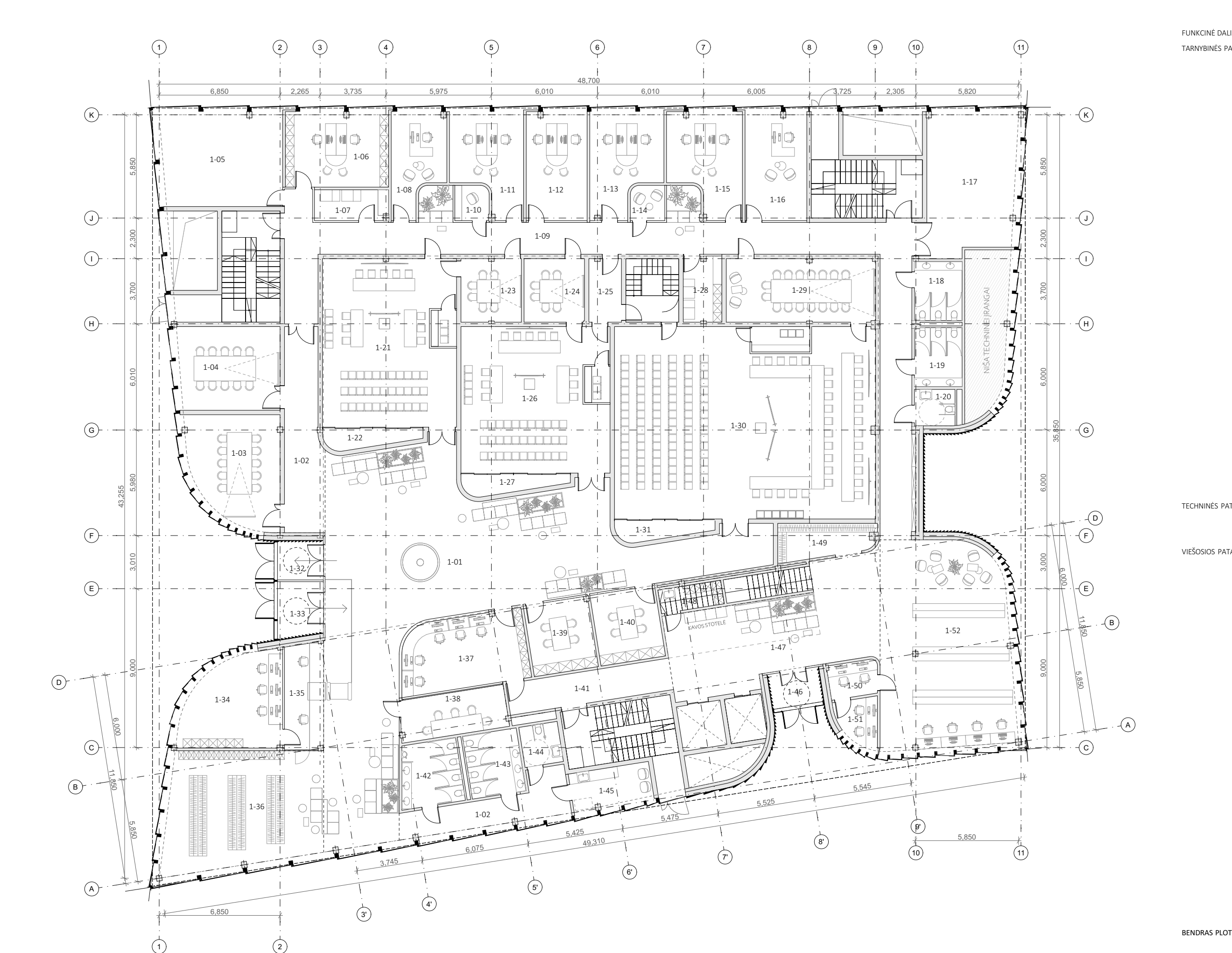
1 AUKŠTO PLANAS M1:200
